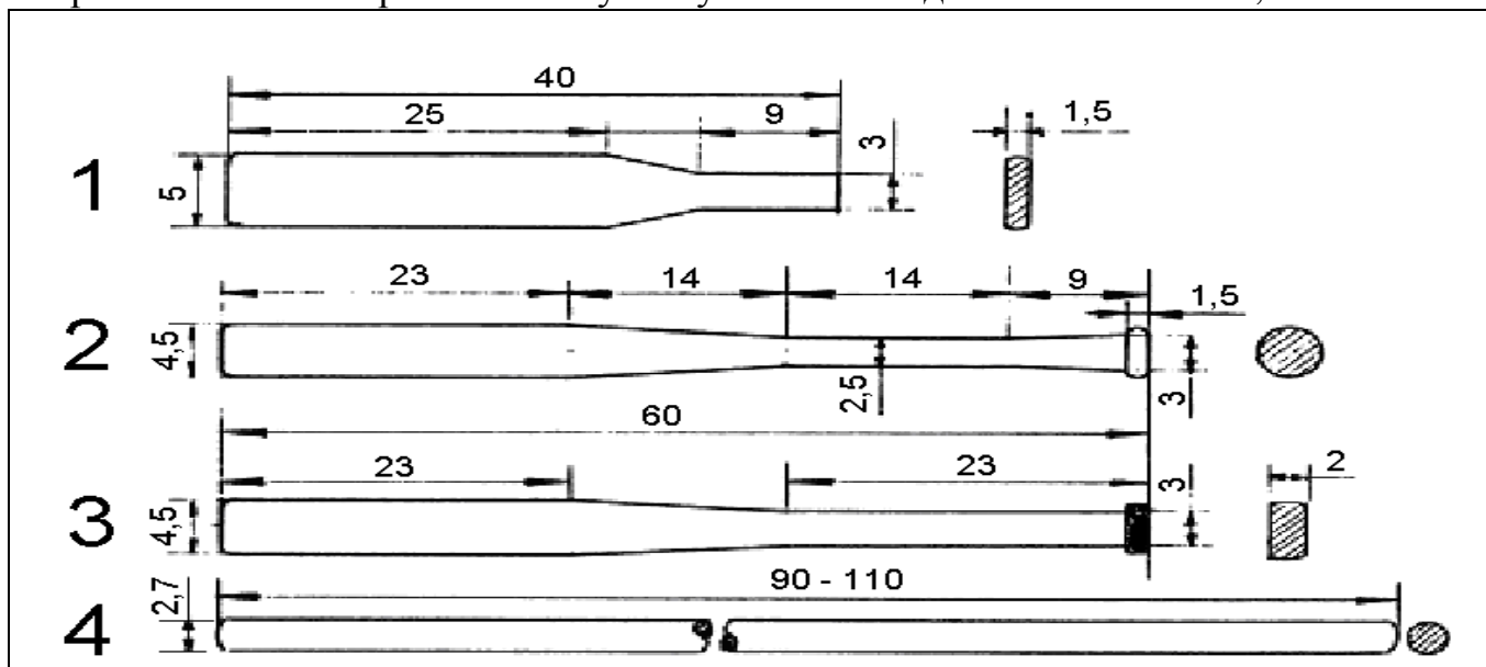
Рис. 84 Размеры бит
