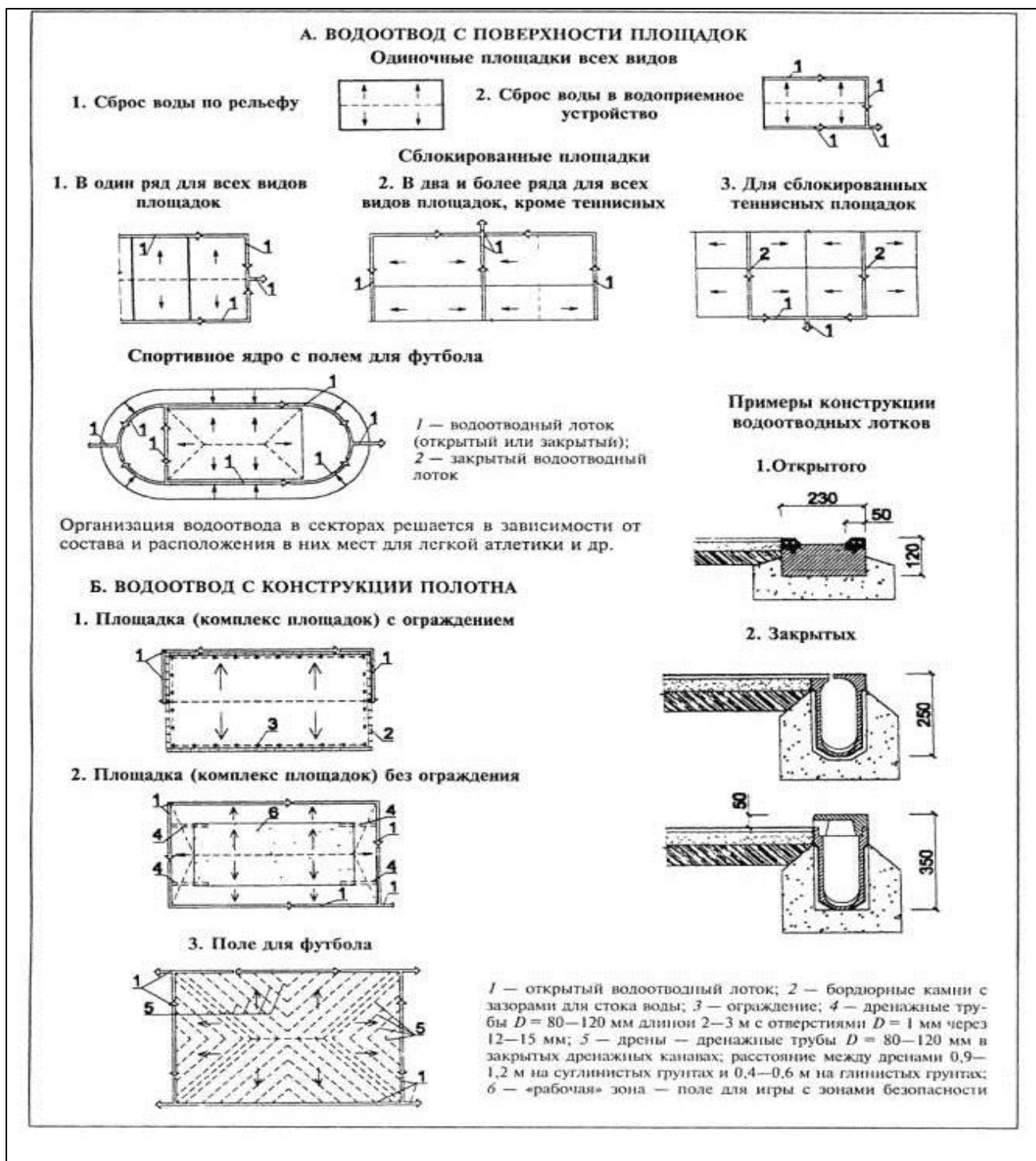
Рис. 29 Схема водоотвода
